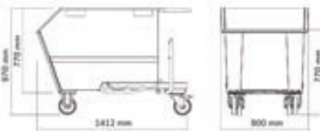
Benna portarottami ribaltabile capacità 500 L con ruote predisposta per griglia e rubinetto
