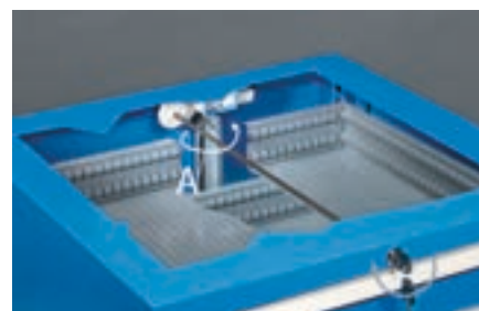
Portata cassetto 50 - 100 kg
