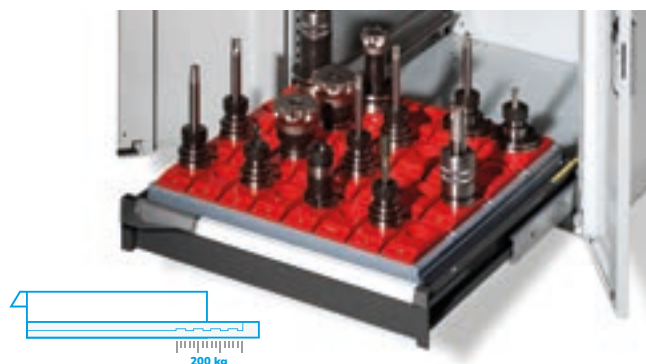
GUIDA TELESCOPICA CONFIGURATA PER ESTRAZIONE TOTALE 200 KG
