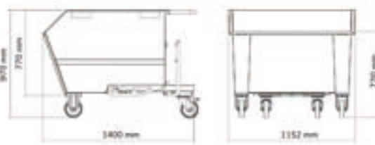
Benna portarottami ribaltabile capacità 750 L con ruote predisposta per griglia e rubinetto
